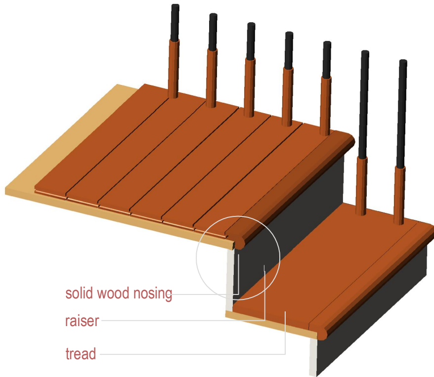
Fig. 12a Nosing
